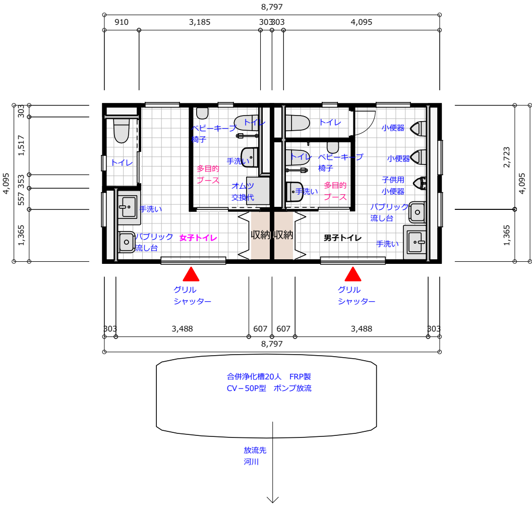
1 階 縮尺 1/100
